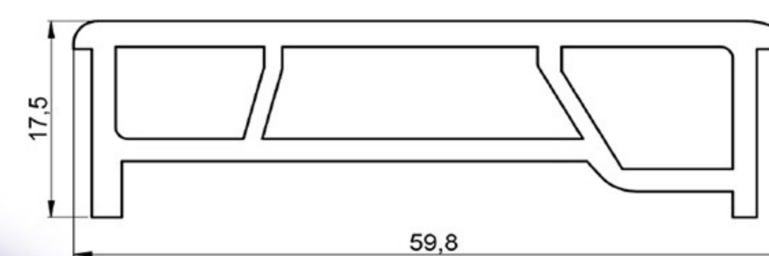
REFRIGERATOR DOOR FRAME
